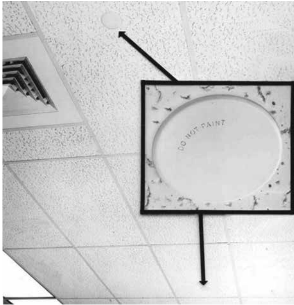
Figura 41 – Bico Oculto não Ferroso em Forro
